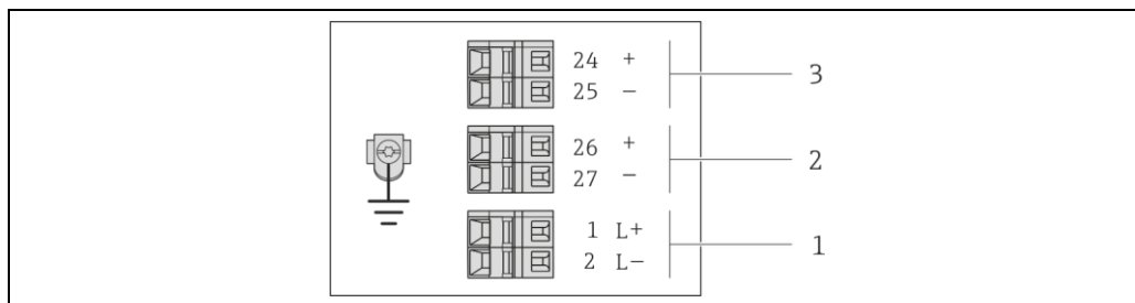
8 Назначение контактов: 4...20 мА HART с импульсным/частотным/релейным выходом
