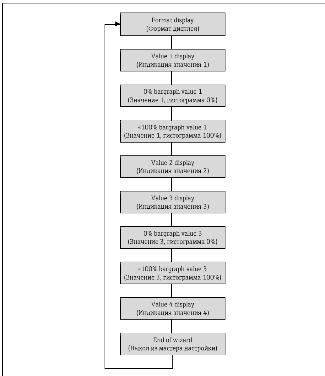
14 Мастер «Display» (Дисплей) в меню «Setup» (Настройка)
